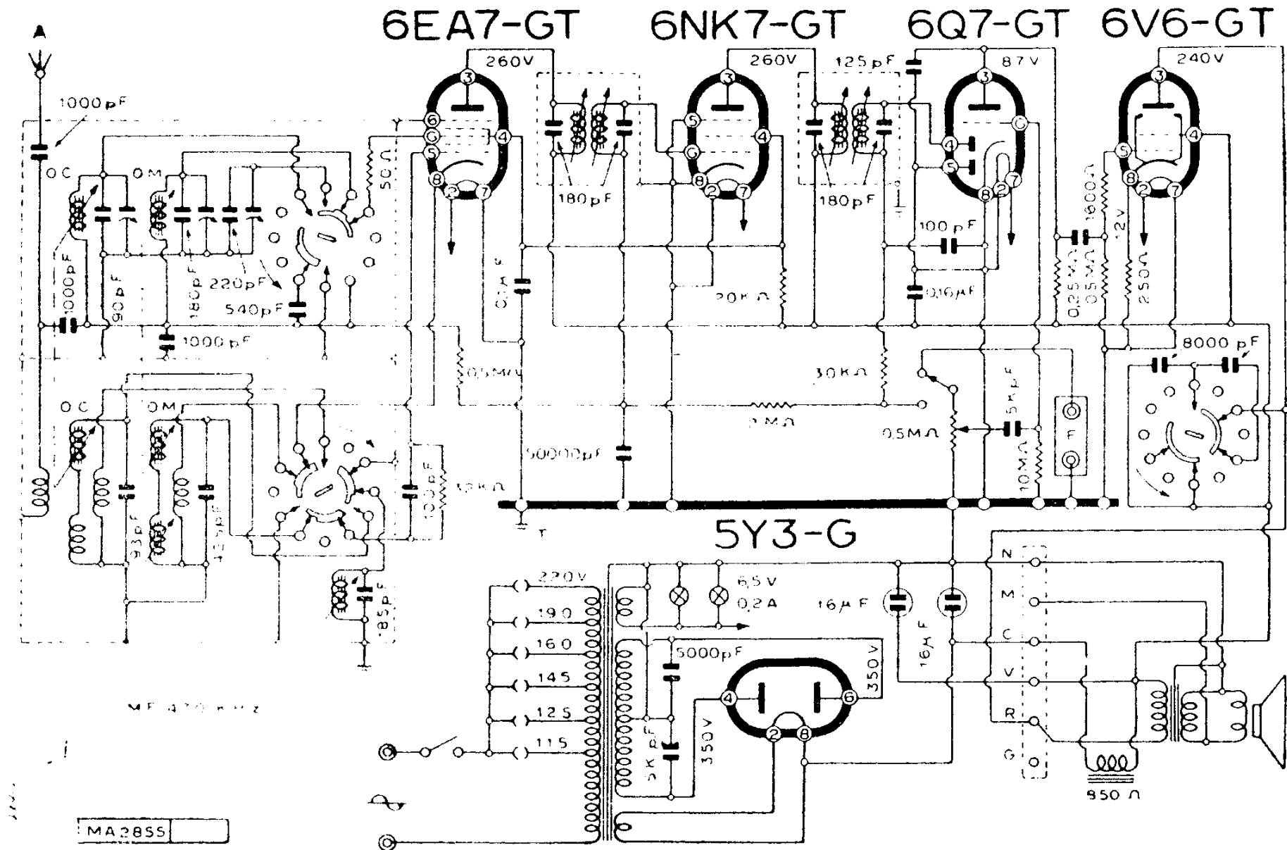
RADIOMARELLI - MOD. « 9A85 »
